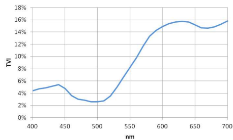
Egy 50%-os cian autotípiai nyomat TVI értékének hullámhosszfüggése
